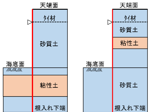
(c) 互層地盤(粘性土主体)
