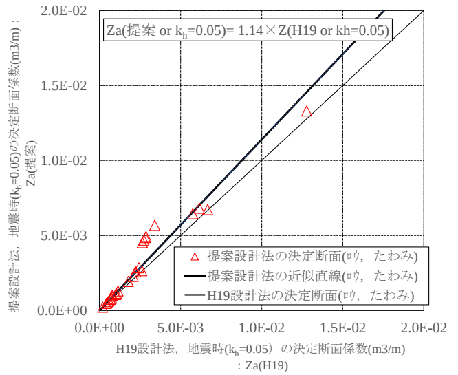
図-6.16 ロウの補正による方法, たわみ曲線法による H19 設計法と提案設計法の地震時( k_h=0.05 )との決定断面
