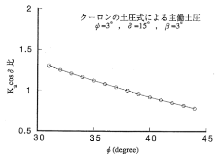
付図A-11 クーロン土圧式による主働土圧 ( \phi の影響) 9)
