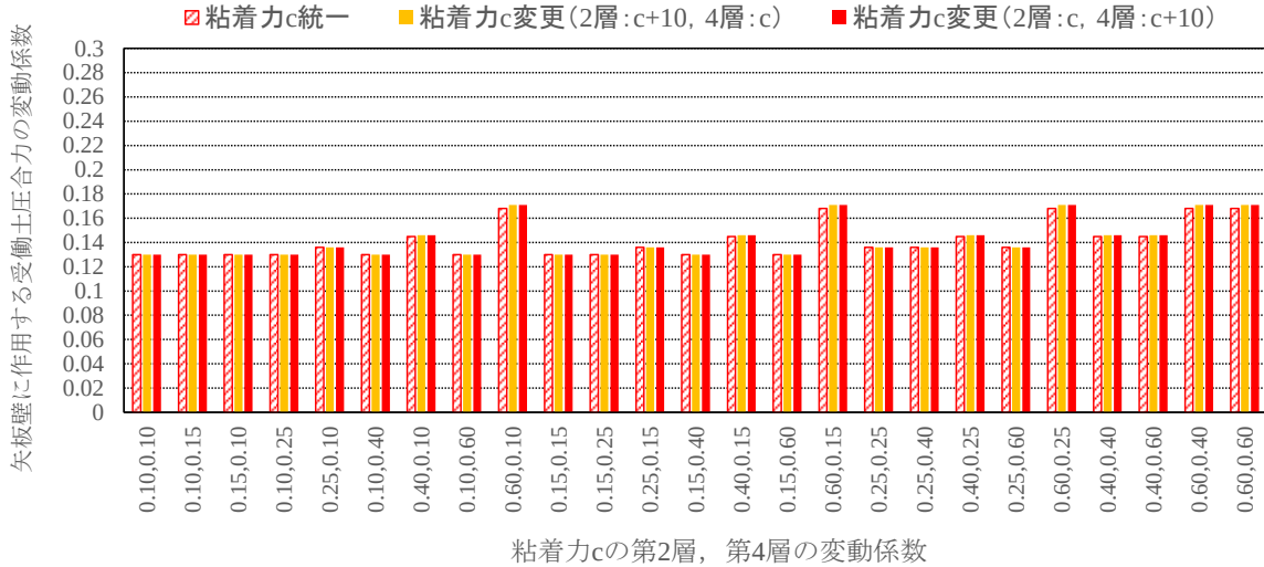
付図 D-18 粘着力 c の大小および変動係数の違いによる矢板壁に作用する受働土圧係数 (全体平均)
