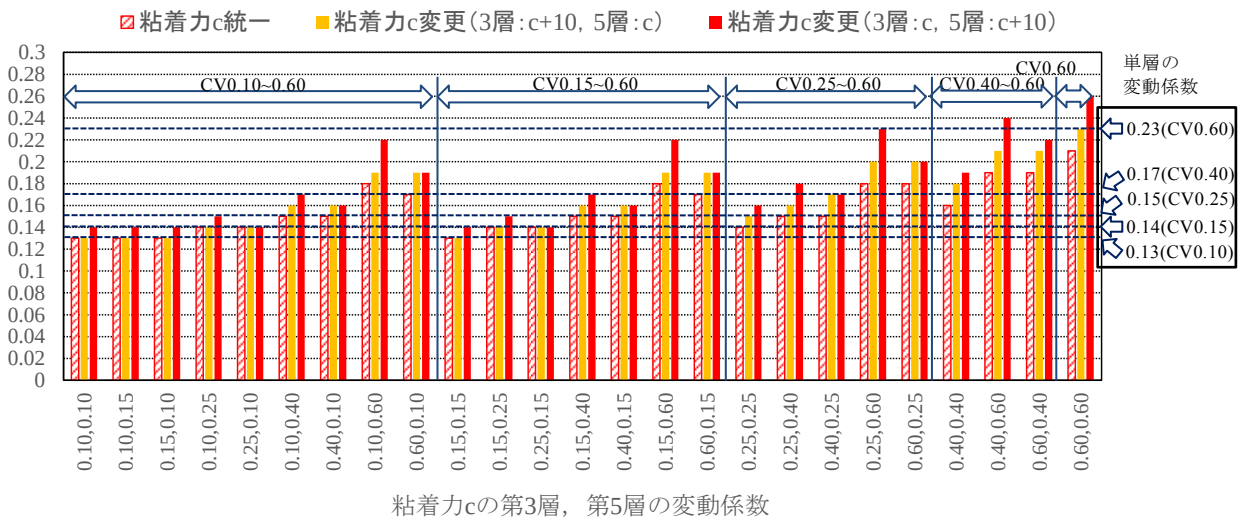
付図 D-16 粘着力 c の大小および変動係数の違いによる矢板壁に作用する主働土圧係数 (粘性土主体)
