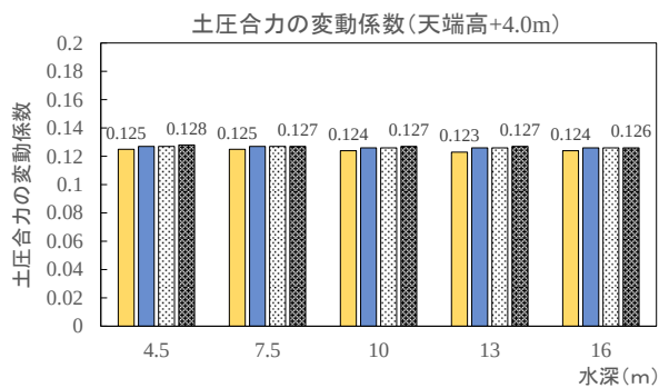
■ ケース1 \phi 30^\circ 単層 ■ ケース2 \phi 40^\circ 単層 □ ケース3 \phi 30^\circ - \phi 40^\circ 2層 ■ ケース4 \phi 30^\circ - \phi 35^\circ - \phi 40^\circ 3層
