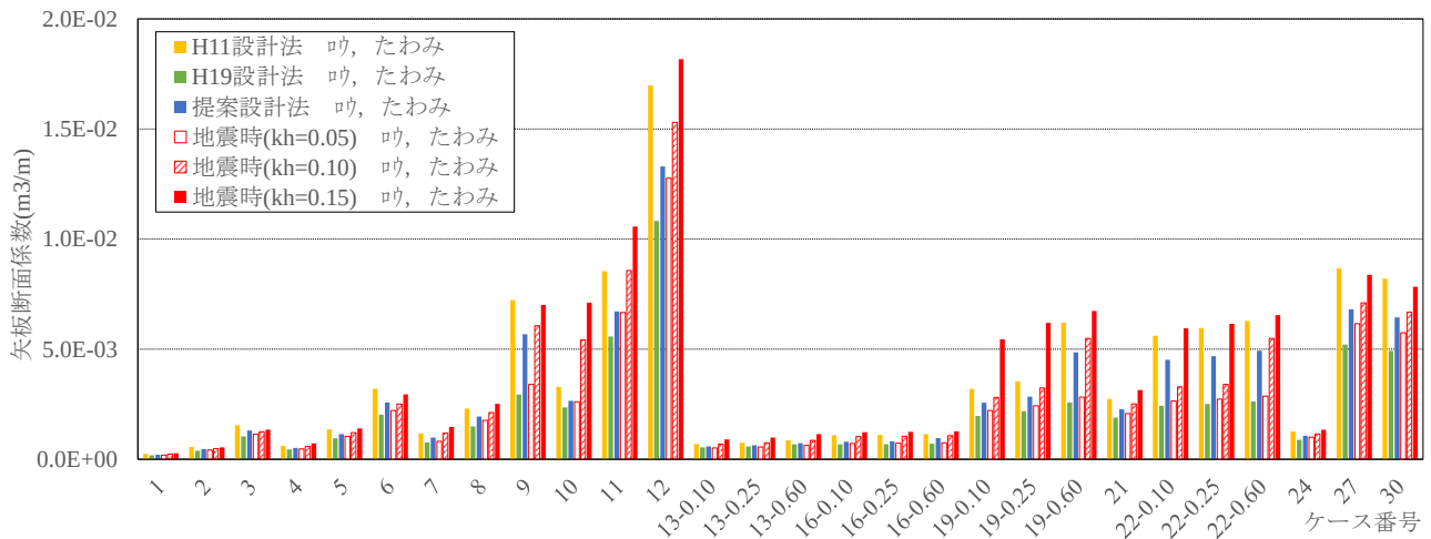
図-6.12 ロウの補正による方法，たわみ曲線法による矢板断面係数
