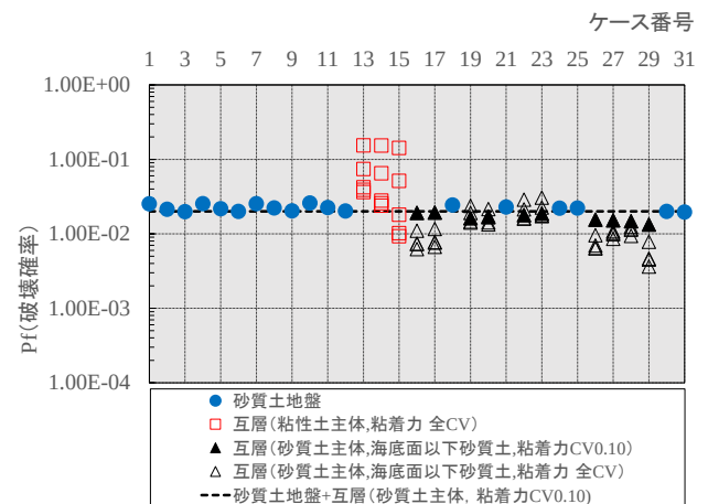
図-4.18 目標破壊確率の設定（根入れ長）
