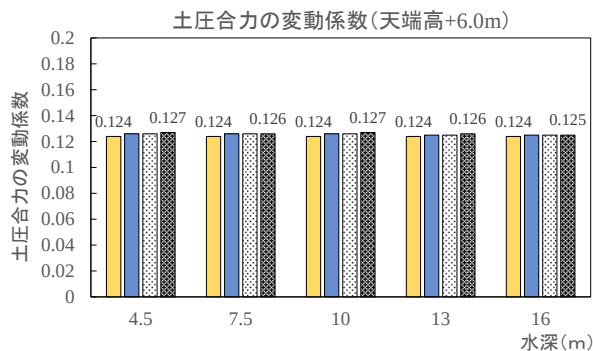
■ ケース1 \phi 30^\circ 単層 ■ ケース2 \phi 40^\circ 単層 □ ケース3 \phi 30^\circ - \phi 40^\circ 2層 ■ ケース4 \phi 30^\circ - \phi 35^\circ - \phi 40^\circ 3層
