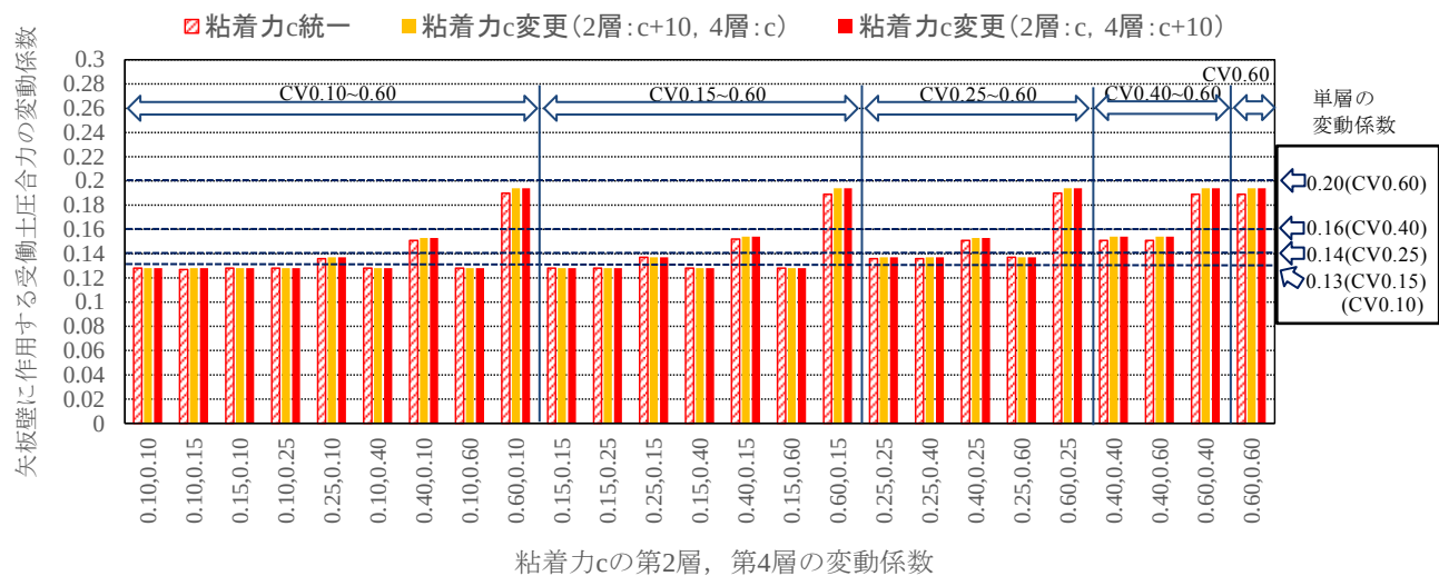
付図 D-20 粘着力 c の大小および変動係数の違いによる矢板壁に作用する受働土圧係数 (粘性土主体)
