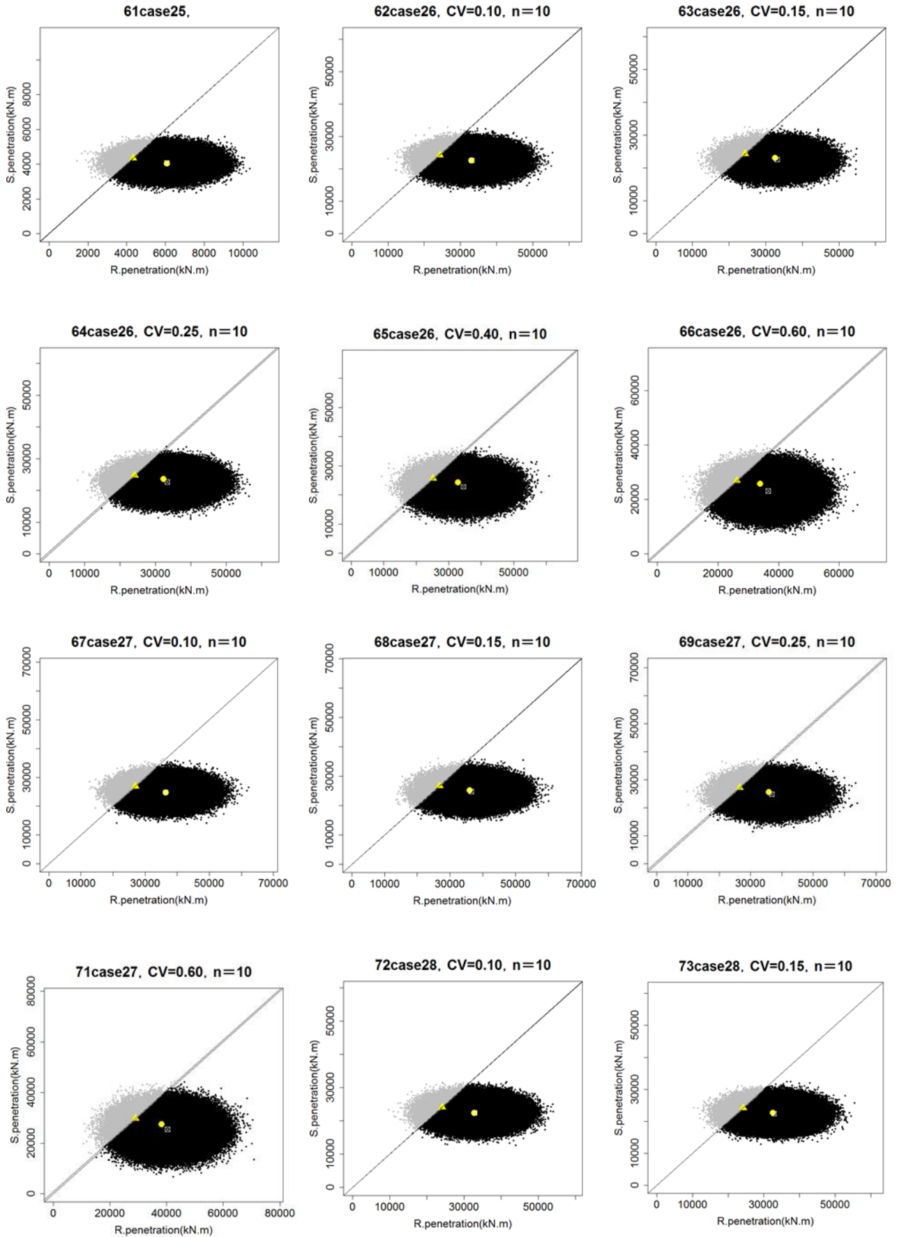
付図 G-6 根入れ長の MCS 図 (6/7)
