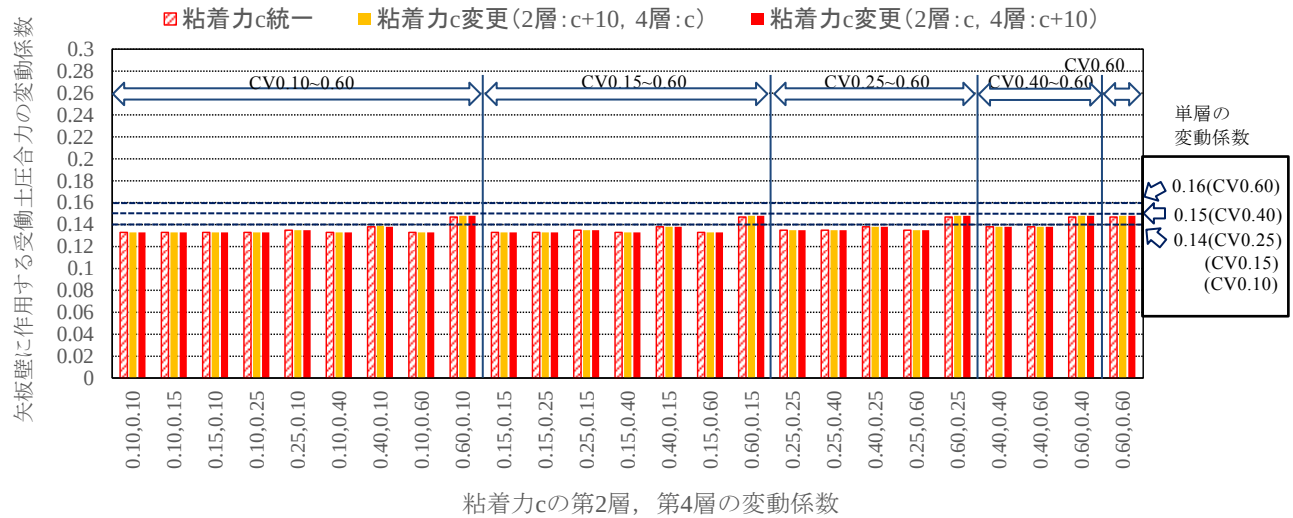
付図 D-19 粘着力 c の大小および変動係数の違いによる矢板壁に作用する受働土圧係数 (砂質土主体)
