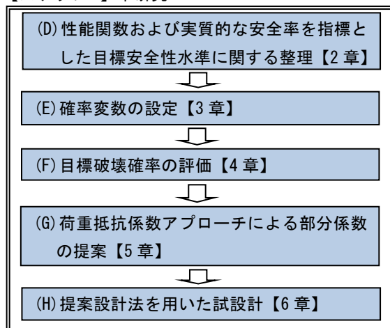
図-1.1 控え矢板式係船岸の永続状態におけるレベル1信頼性設計法に関する部分係数の設定フロー
