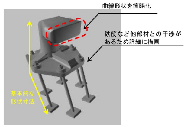
図-3.9 係船柱
