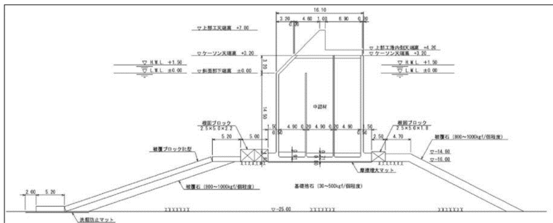
図-3.6 久慈港湾地区防波堤(北堤)
