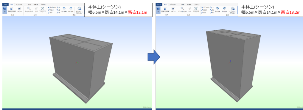
図-3.12 本体工(ケーソン)のパラメトリック化
