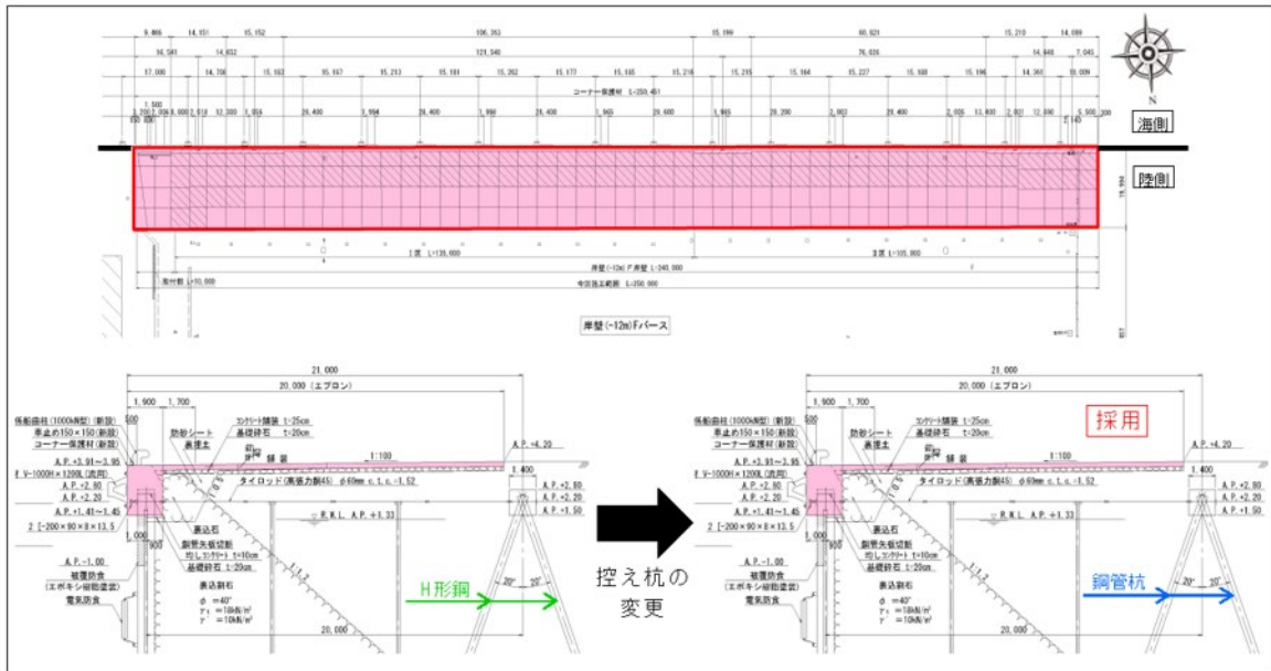
図-3.4 千葉港千葉中央地区岸壁
