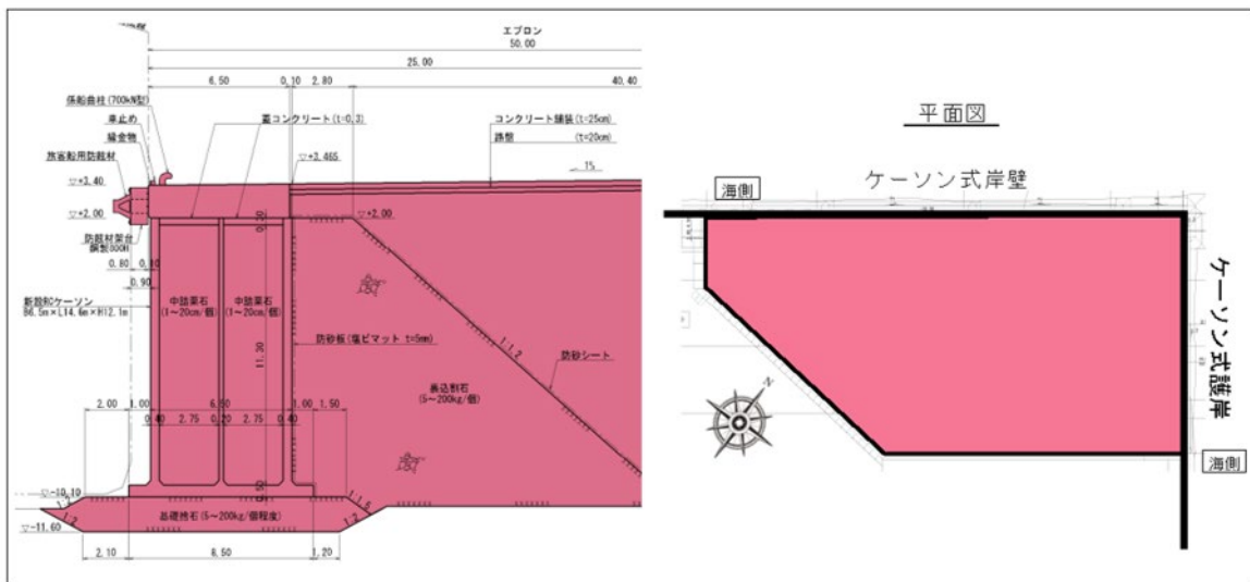
図-3.5 平良港漲水地区岸壁
