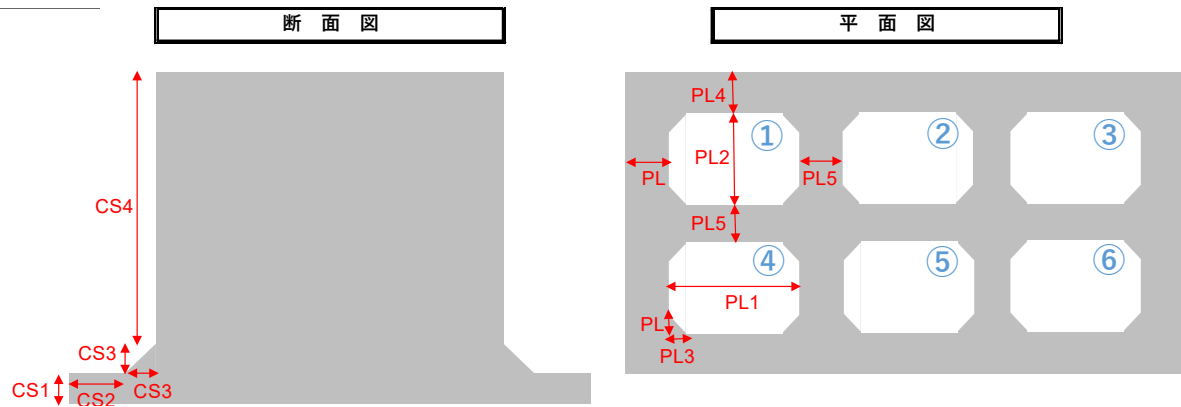
図-3.11 本体工(ケーソン)コントロール画面
