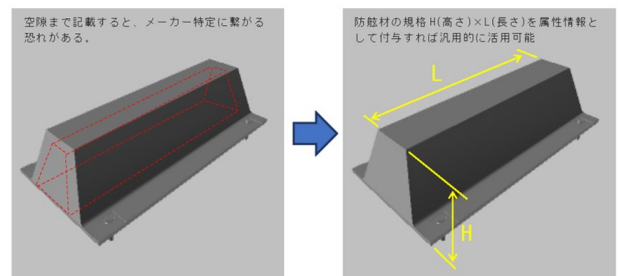
図-3.10 防舷材
