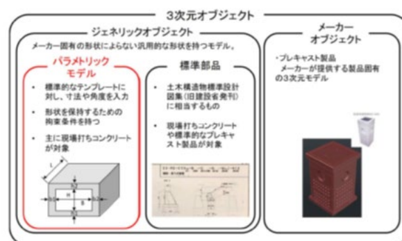
図-3.2 3次元モデルの分類
