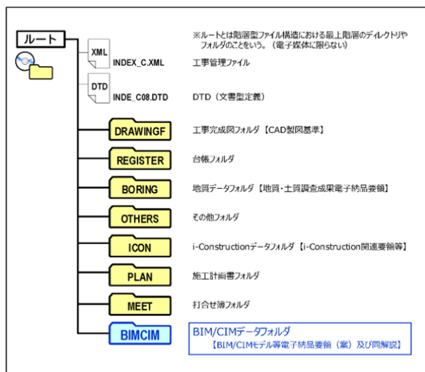
図-2.2 工事完成図書の電子成果品のフォルダ構成 3)
