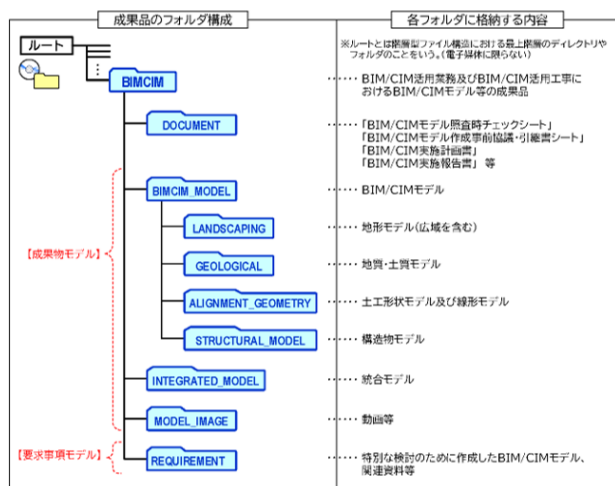
図-2.3 BIM/CIMモデル等の成果品フォルダ構成 3)
