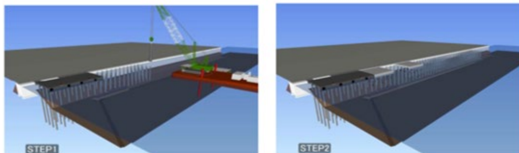
作成したモデルの施工手順図への活用
